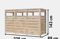
3ER MÜLLTONNEN-UNTERSTAND Seite 63
