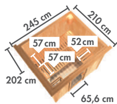
Abb. MALIN mit bronzierter Ganzglastür und Zubehör (gegen Aufpreis): Sternenhimmel
