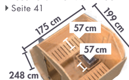
FASSSAUNA ASYMMETRISCH 1 ▶ Seite 41
