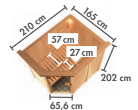
Zeichnung und Maße mit Dachkranz
