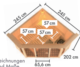
Abb. ALCINDA mit Dachkranz, bronzierter Ganzglastür Classic und Zubehör (gegen Aufpreis): Saunaleuchte Modern
